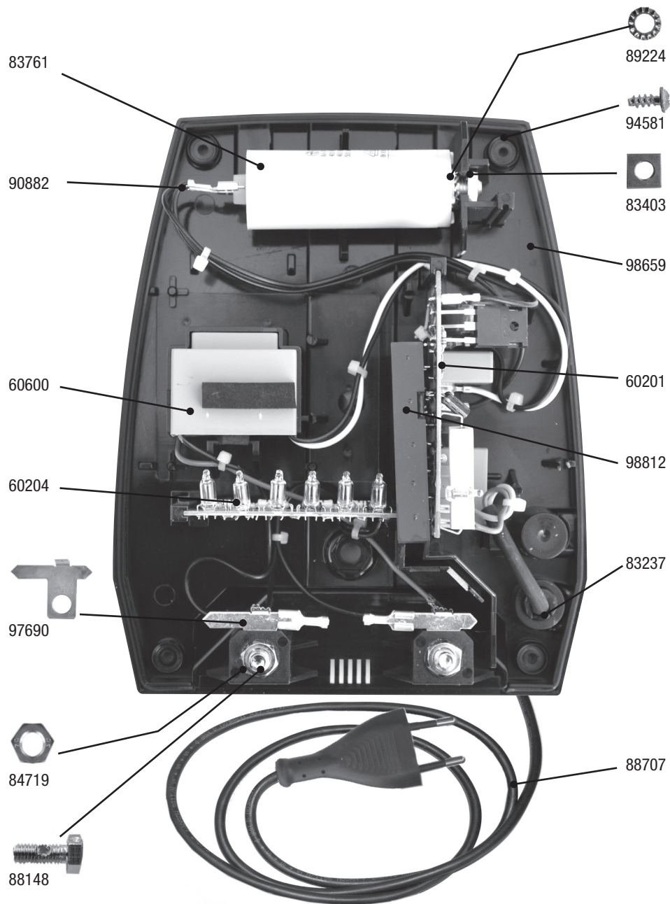
Fig. 1 Ersatzteile | Spare parts | Pièces détachées | Peças | Pezzi di ricambio Reservevedele | Reserve onderdelen | Náhradné diely
