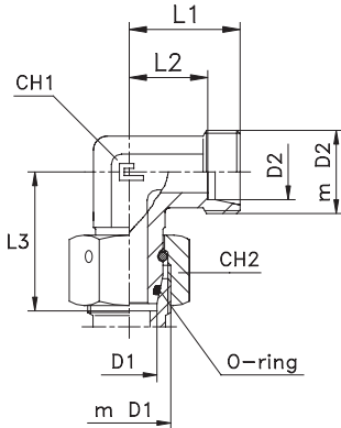
Typ: 6042...1 Körper
