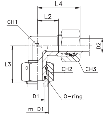
Typ: 6042...4 Ring B4
