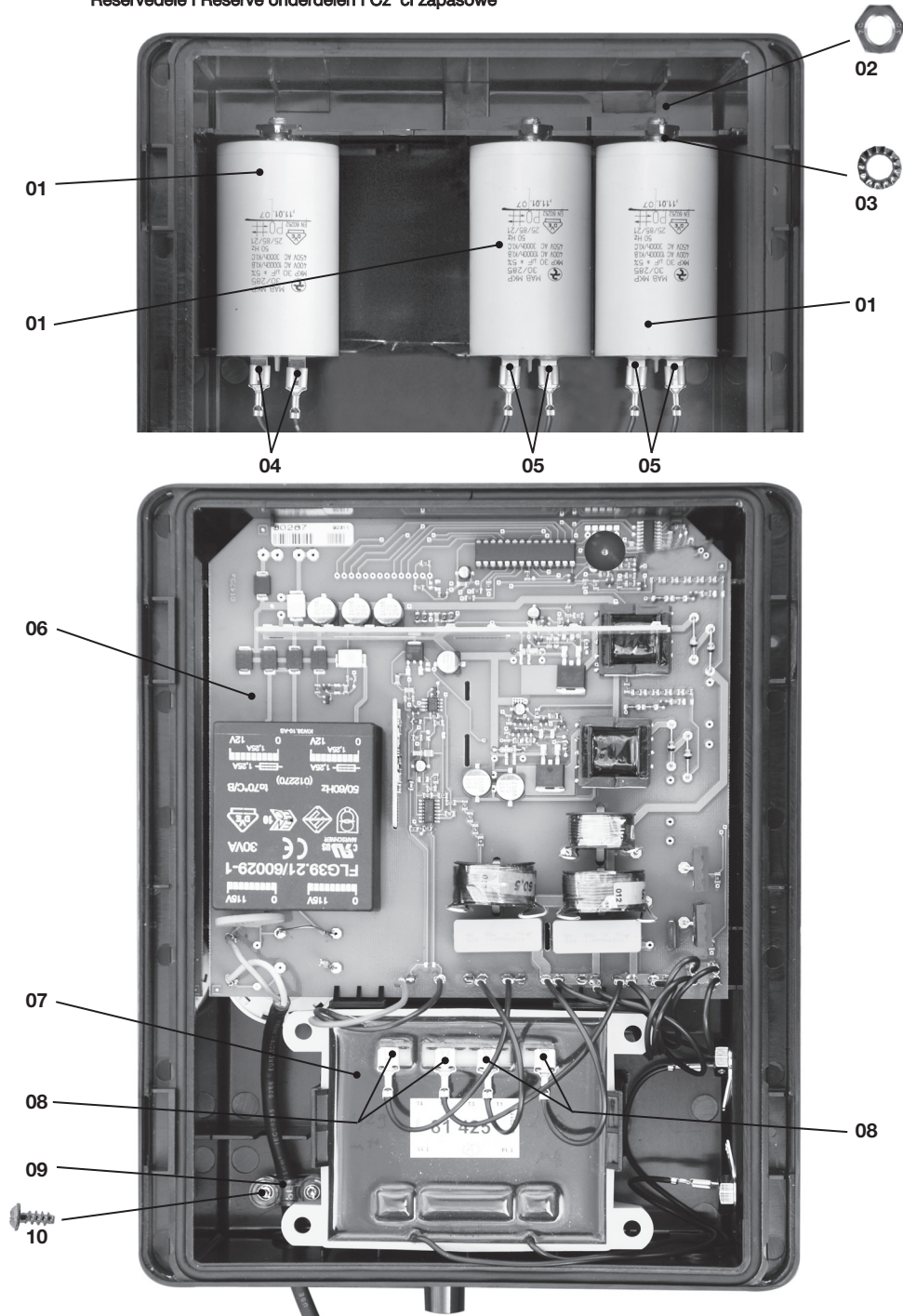
Fig. 1 Ersatzteile | Spare parts | Pièces détachées | Peças | Pezzi di ricambio | Reserveedele | Reserve onderdelen | Cz ci zapasowe
