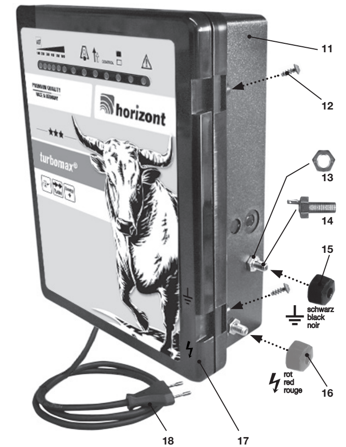
Fig. 2 Ersatzteile | Spare parts | Pièces détachées | Peças | Pezzi di ricambio | Reserveedele | Reserve onderdelen | Cz ci zapasowe
